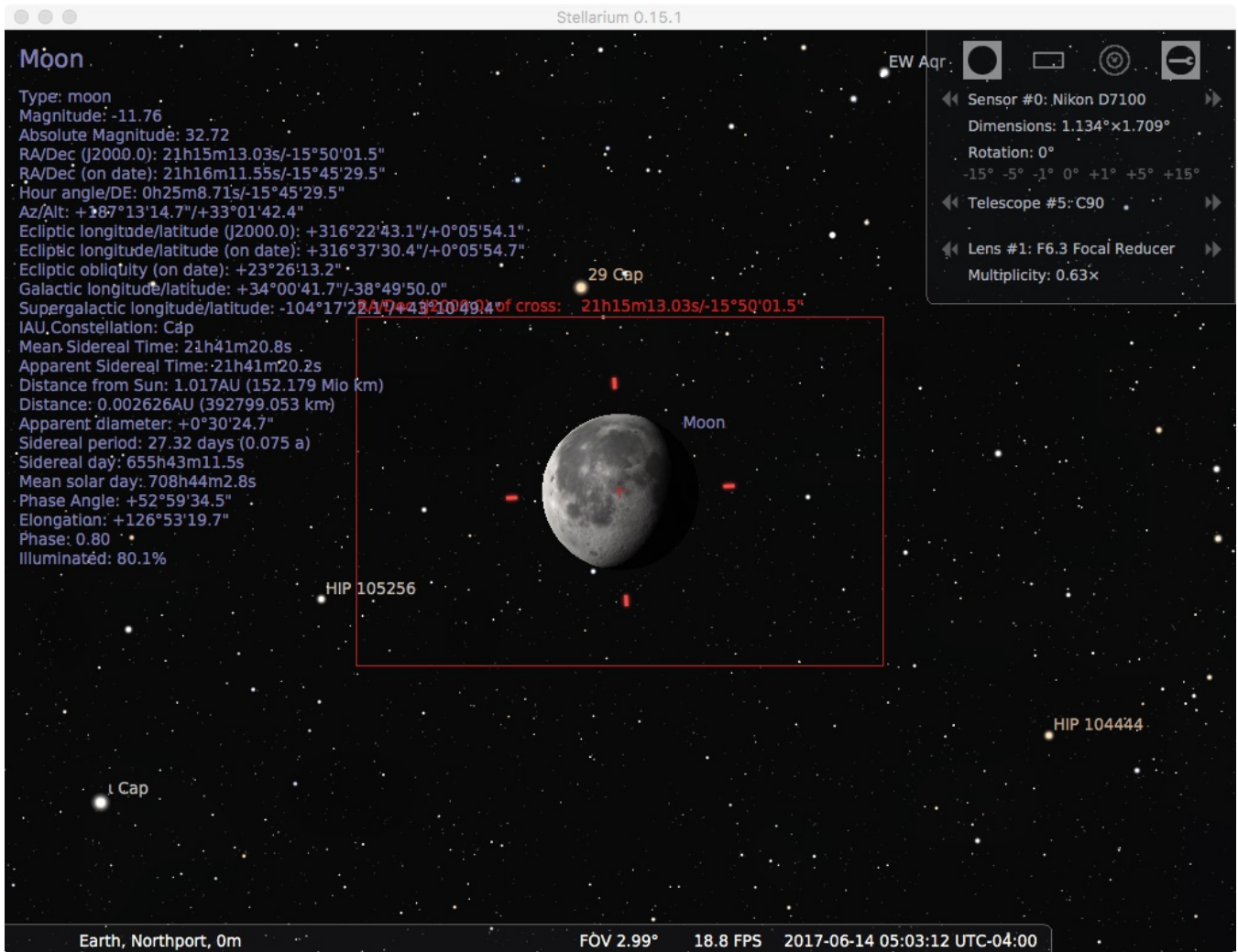
Moon - APS-C, 1250 mm FL FR.63 Telescope
